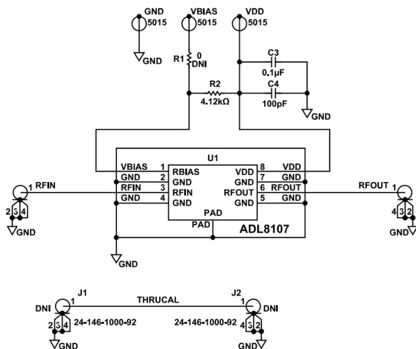
Figure 4. ADL8107-EVALZ Schematic
