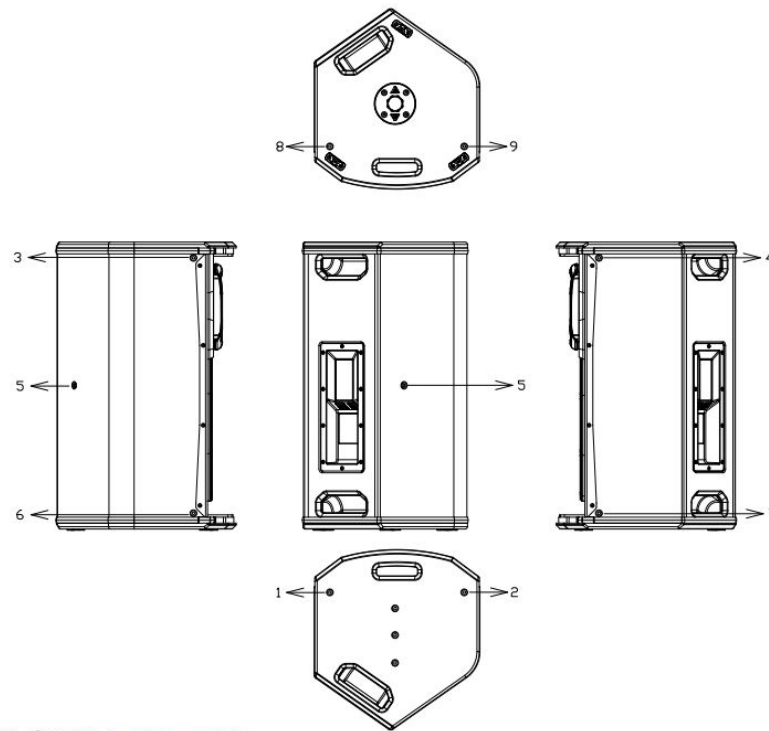
Fig. 18. S15P rigging points
