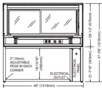
ED2SYS-48/2S
