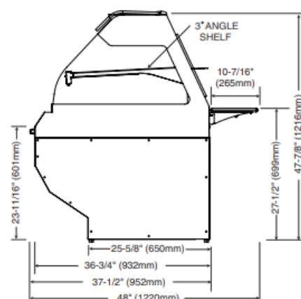
ED2SYS-2S PROFILE
