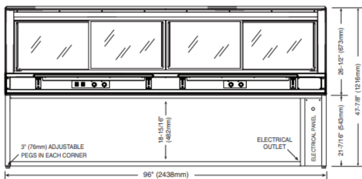
ED2SYS-96/2S
