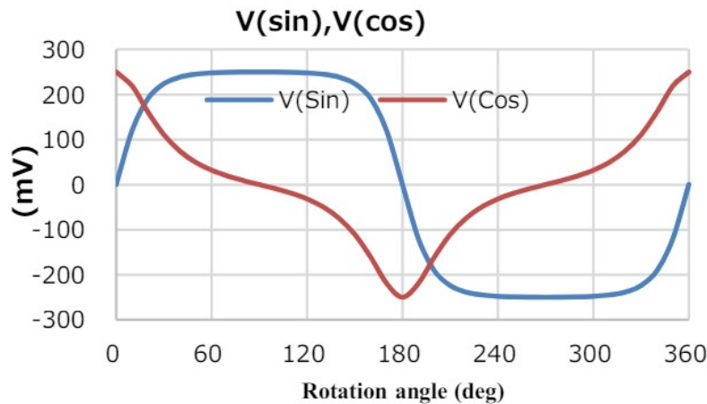
Fig. 15 Sensor output
