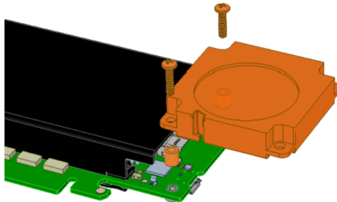
Figure 5 : ADM-PCIE-9H3 Fan Assembly
