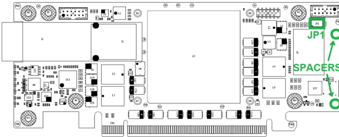
Figure 4 : ADM-PCIE-9H3 Fan Plug
