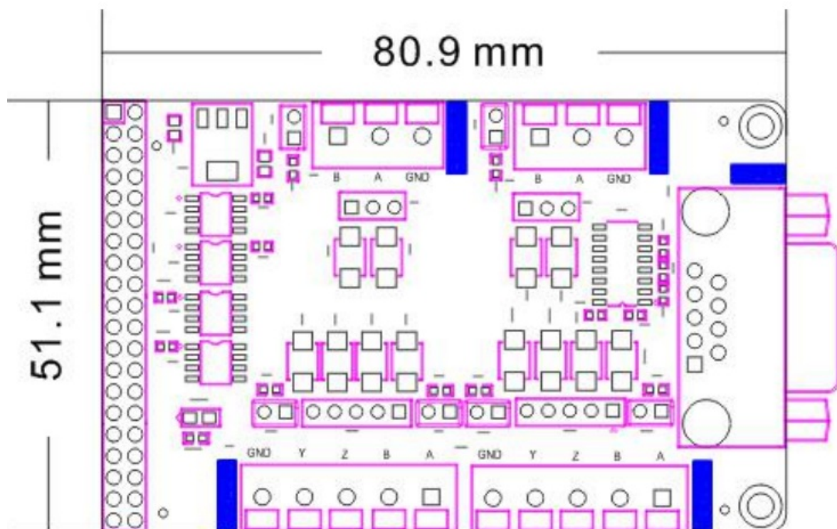
Figure 1-2: AN3485 Module Size Dimension
