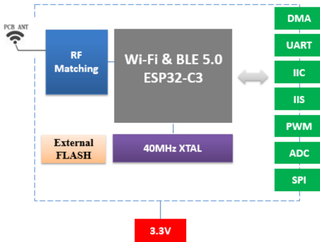
Fig.1.1 ESP-C20 Module Structure
