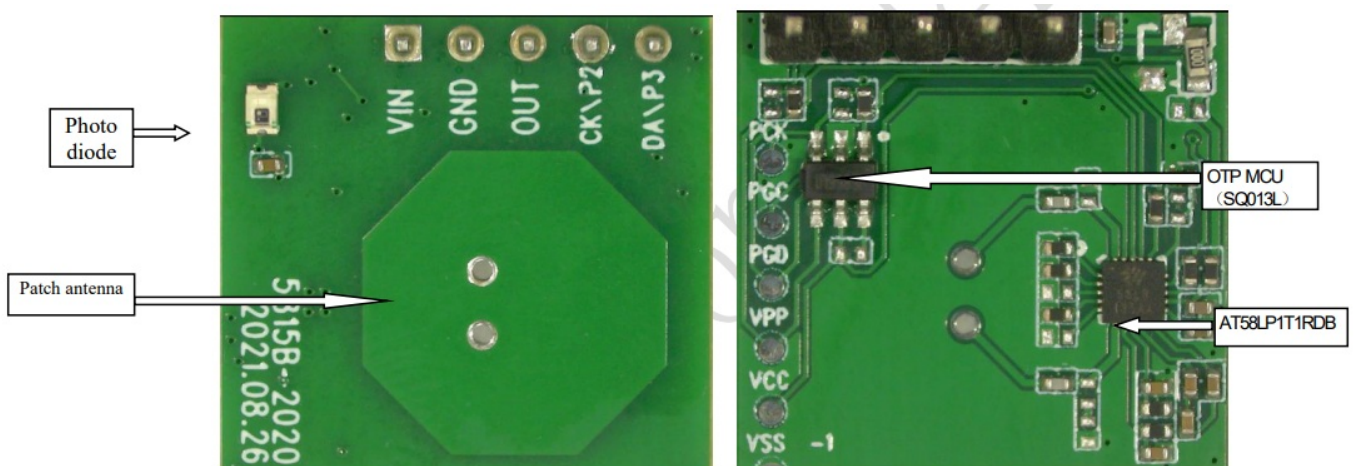
Plot. 1 AT58L4LDB-2020 module
