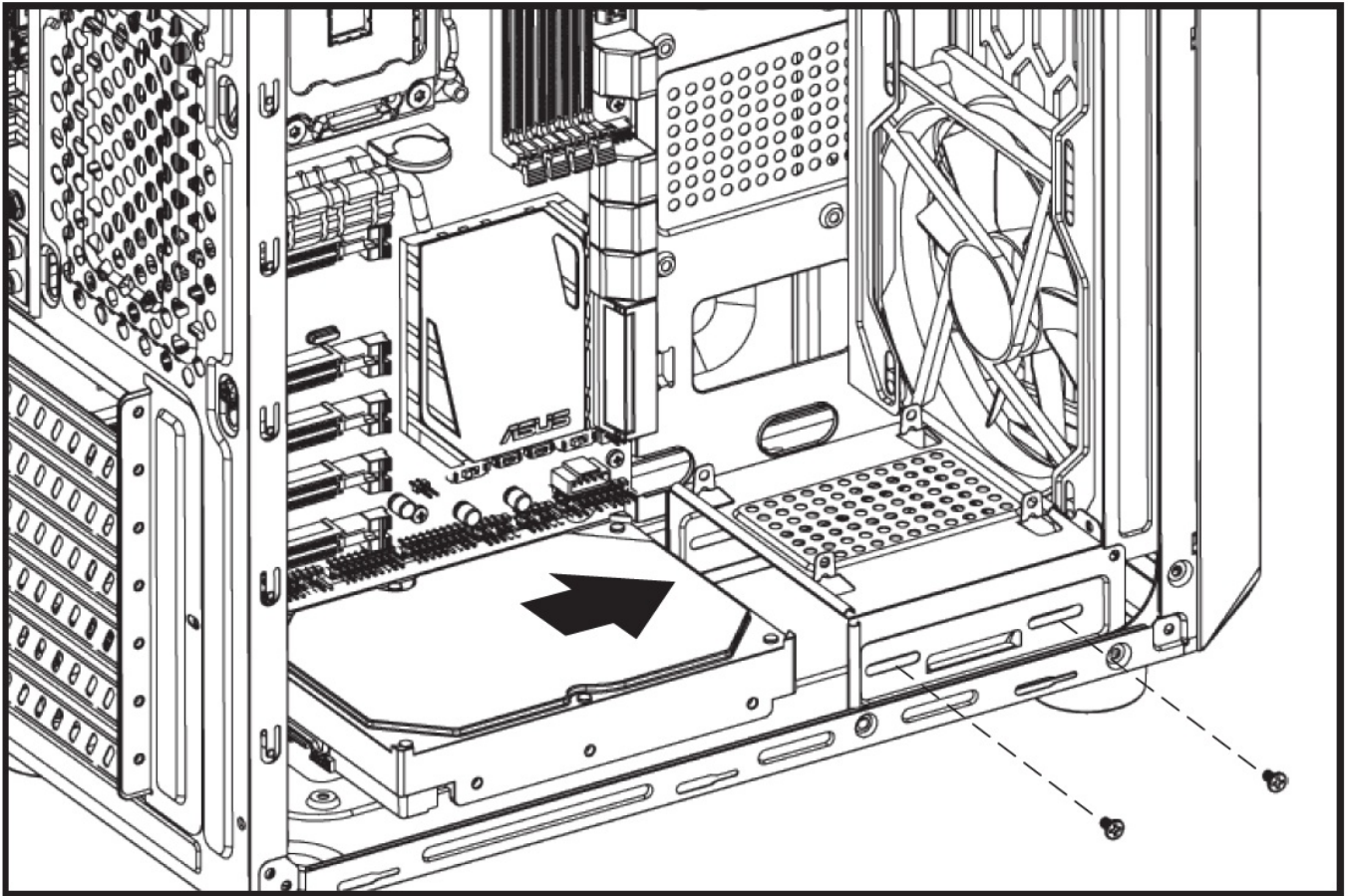
2.5" HDDx4
