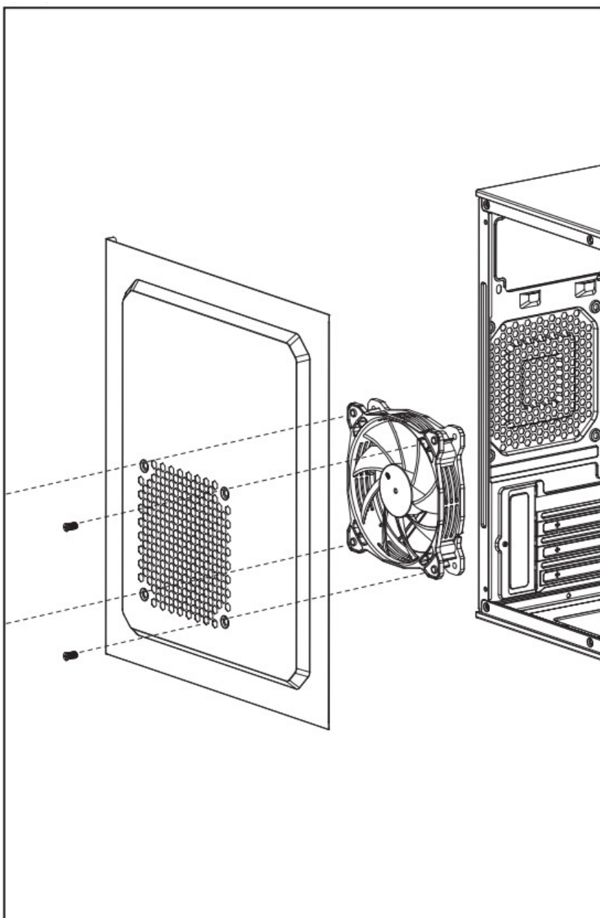
Install Fan
