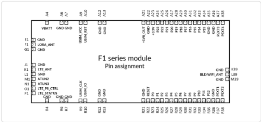
Figure 3: F1 Smart Module Pin-out (Top View)
