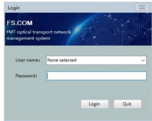
Fig.4.8 Login
