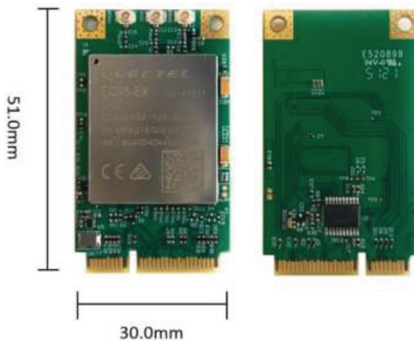
Figure 1. miniPCIe EG95 LTE Cat 4 module.
